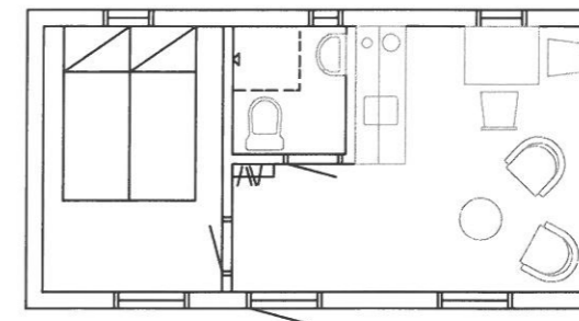
PLAN MÖBLERAD
